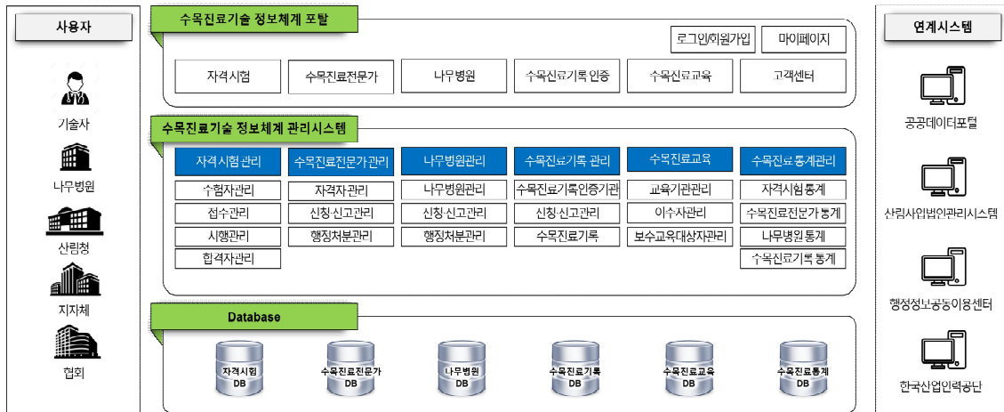
[그림 1] 수목진료기술 정보체계 구성(안)
