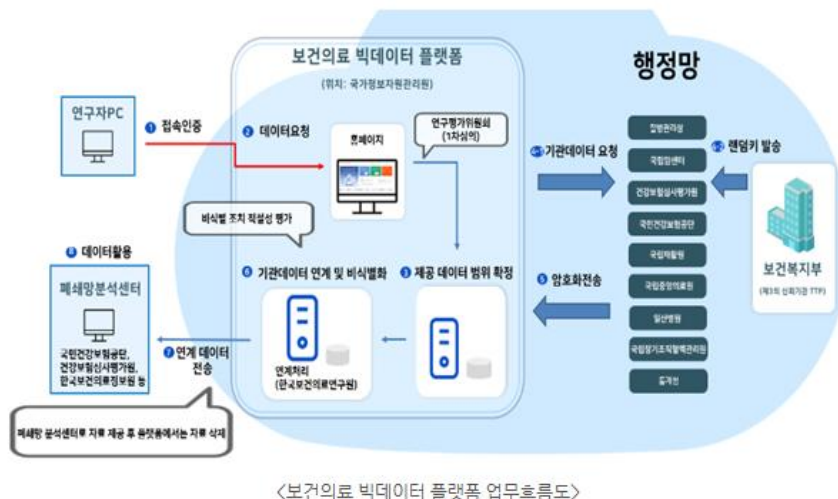
<보건의료 빅데이터 플랫폼 업무흐름도>
